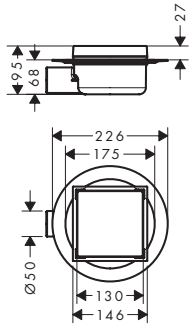
RainDrain Spot Rost rückseitig befliesbar
