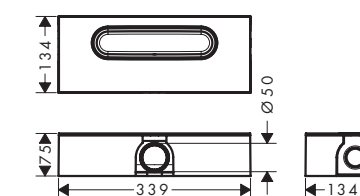
uBox universal für Standardinstallation
