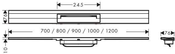
RainDrain Flex mit Wandmontage
