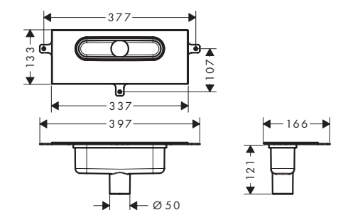
uBox universal für vertikale Installation
