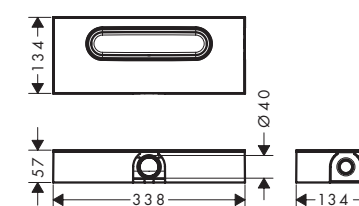
uBox universal für flache Installation
